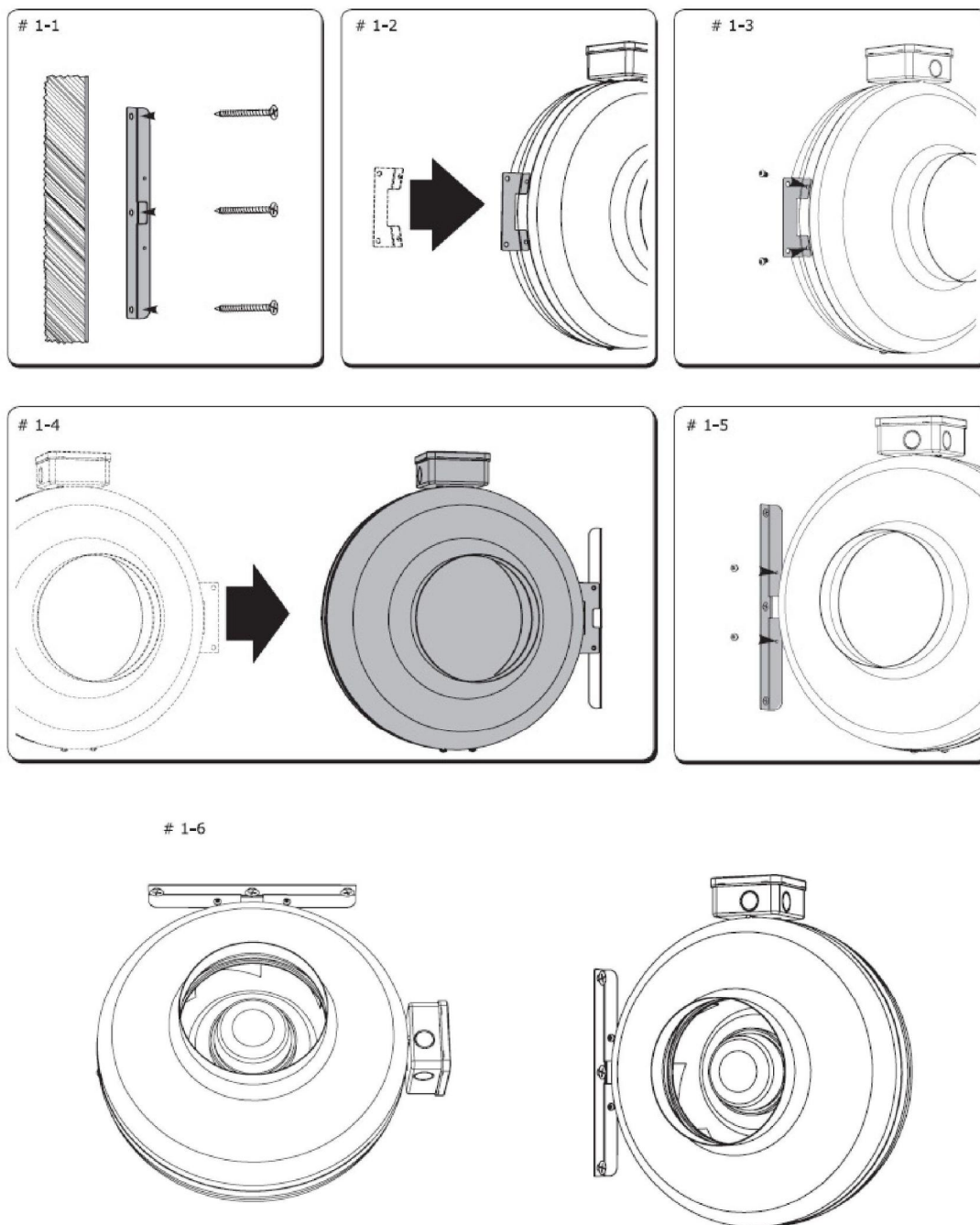
1. ábra - Készülék fali rögzítése tartószerkezettel
