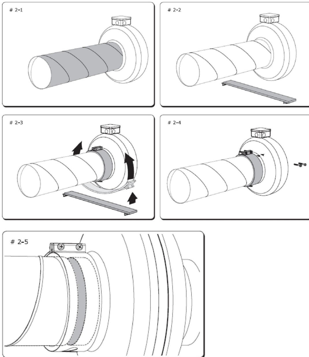
2. ábra - Csatlakoztatás légcatornához rezgéstompító rögzítőbilincs használatával
